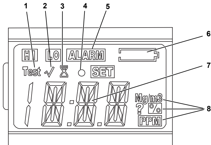
Рис. 2 Дисплей
